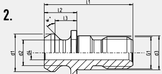
2. ISO 7388-3 Form UD mit Durchgangsbohrung /with drill through (ehemalige Norm /previous norm DIN 7388-2 Form B)
